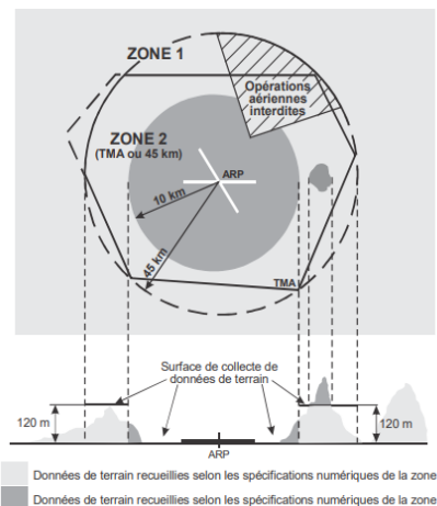
Figure A8-1. Surfaces de collecte de données de terrain — Zones 1 et 2
